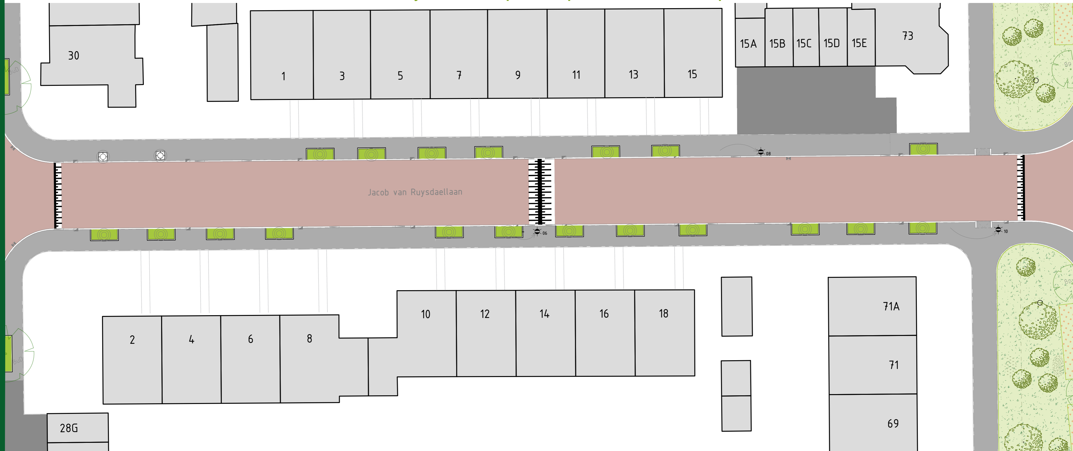
OVERZICHTSTEKING SCHAAL 1:200
